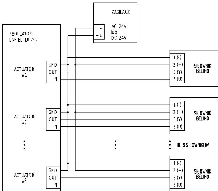
Rysunek 3.7: Schemat podłączenia siłowników analogowych Belimo
