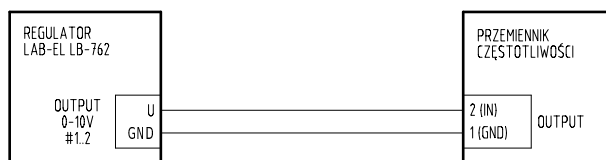
Rysunek 3.11: Schemat podłączenia przetwornika częstotliwości typu OBRUSN PC3., OBRUSN PC4., SSD Drives 605, SSD Drives 650 i podobnych
