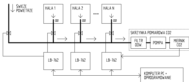
Rysunek 1.6: Schemat układu zbiorczego pomiaru stężenia CO 2
