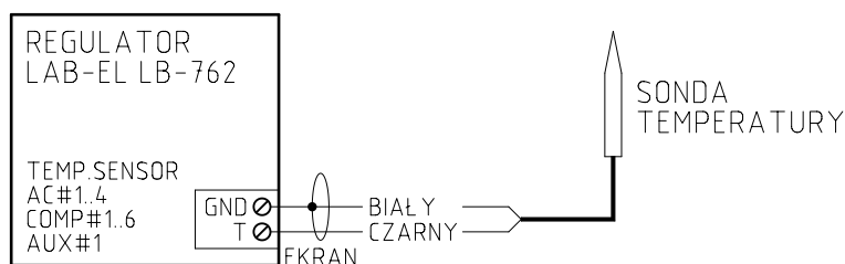
Rysunek 3.2: Schemat podłączenia sondy temperatury
