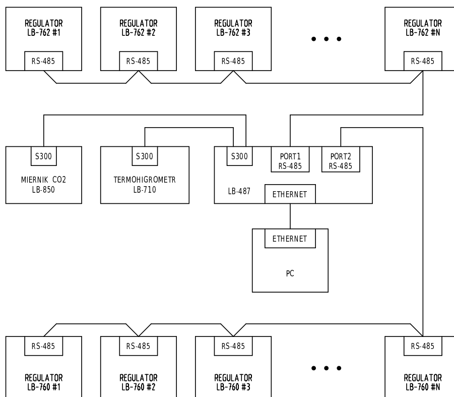
Rysunek 1.5: Schemat systemu z regulatorami LB-762 i LB-760
