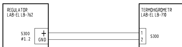
Rysunek 3.5: Schemat podłączenia miernika typu LAB-EL LB-710
