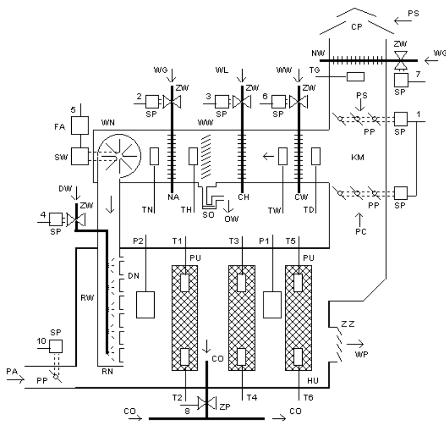
Rysunek 1.2: Urządzenia wykonawcze
