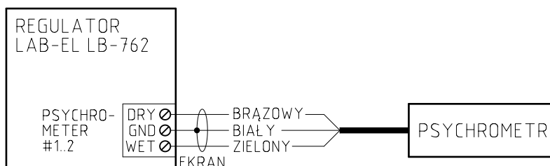
Rysunek 3.1: Schemat podłączenia psychrometru
