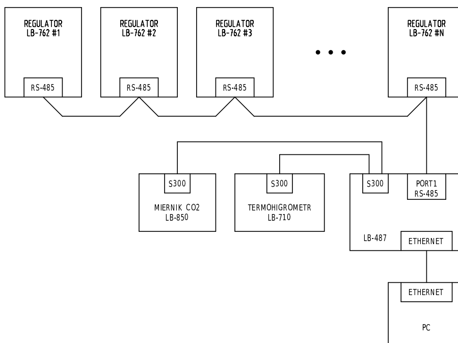
Rysunek 1.4: Schemat systemu z kilkoma regulatorami LB-762 i siecią RS-485
