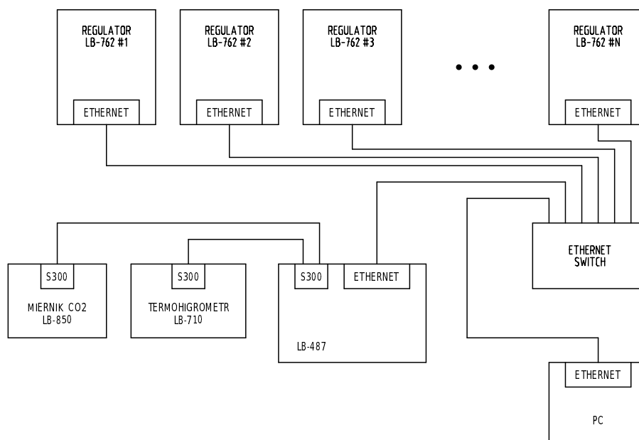
Rysunek 1.3: Schemat systemu z kilkoma regulatorami LB-762 i siecią Ethernet
