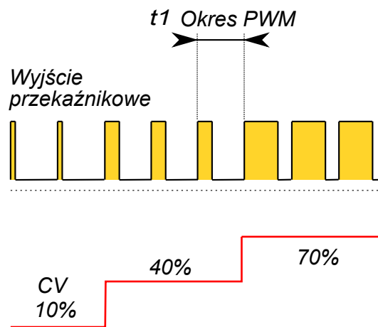
Rysunek 13: Wyjście algorytmu PID – PWM na przekaźniku
