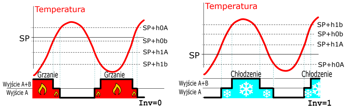
Rysunek 10: Regulacja progowa, opcja 1 – praca z jednym urządzeniem wykonawczym umożliwiającym stopniowanie mocy. Po lewej sterowanie grzałką ( Inv = 0) ; po prawej sterowanie agregatem chłodniczym ( Inv = 1).
