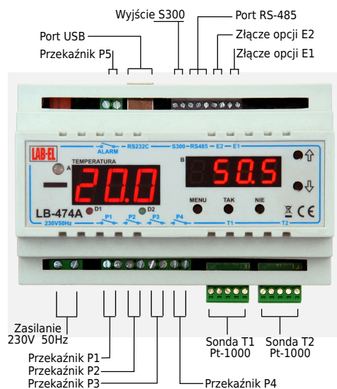
Rysunek 1: LB-474A3 – punkty wejść i wyjść
