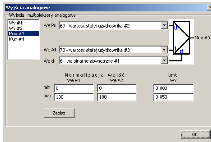
Rysunek 19: Konfiguracja multiplexera #3 w programie ws474.exe
