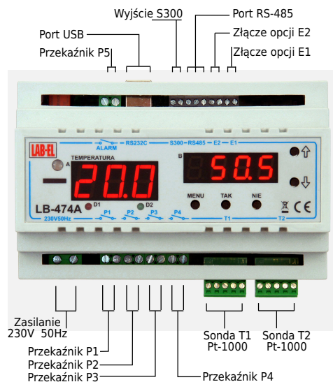
Rysunek 1: LB-474A3 – punkty wejść i wyjść
