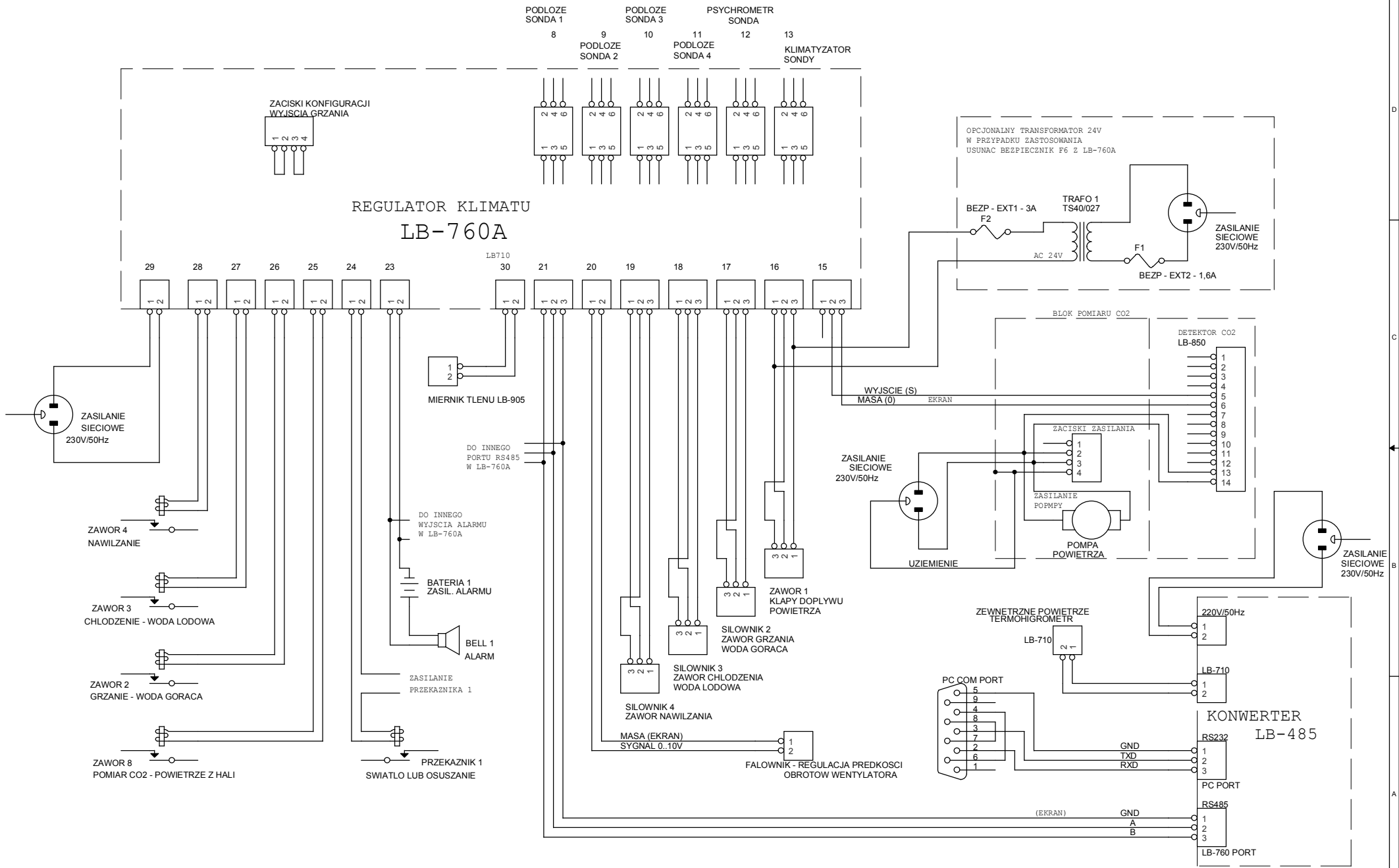
Schemat instalacyjny regulatora klimatu LB-760A z detektorem LB-850
