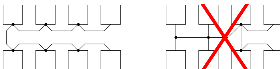
Rysunek 3.13: Schemat prawidłowej i nieprawidłowej topologii sieci RS-485
