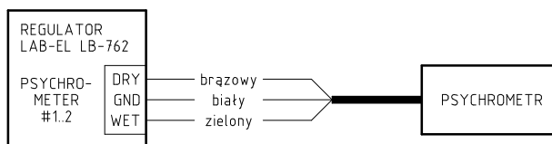
Rysunek 3.1: Schemat podłączenia psychrometru
