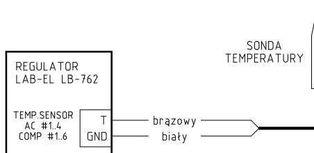
Rysunek 3.2: Schemat podłączenia sondy temperatury
