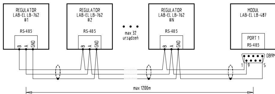
Rysunek 3.13: Schemat połączenia sieci RS-485
