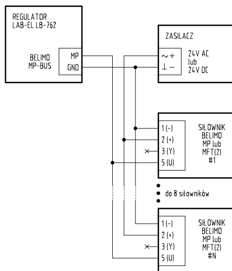
Rysunek 3.11: Schemat podłączenia szyny siłowników BELIMO MP-BUS
