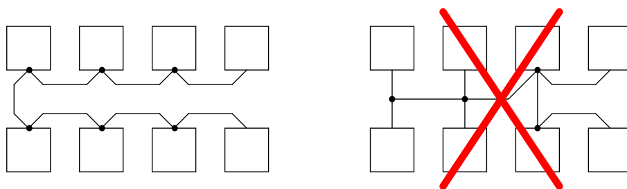
Rysunek 3.14: Schemat prawidłowej i nieprawidłowej topologii sieci RS-485
