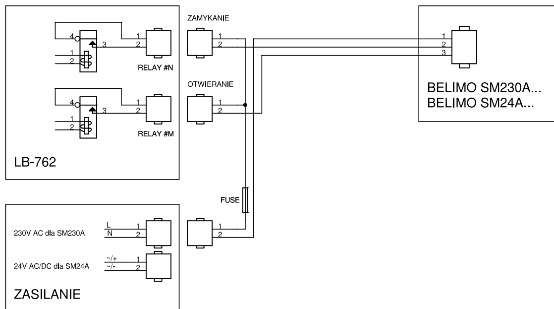
Rysunek 3.10: Schemat podłączenia siłowników typu otwórz-zamknij
