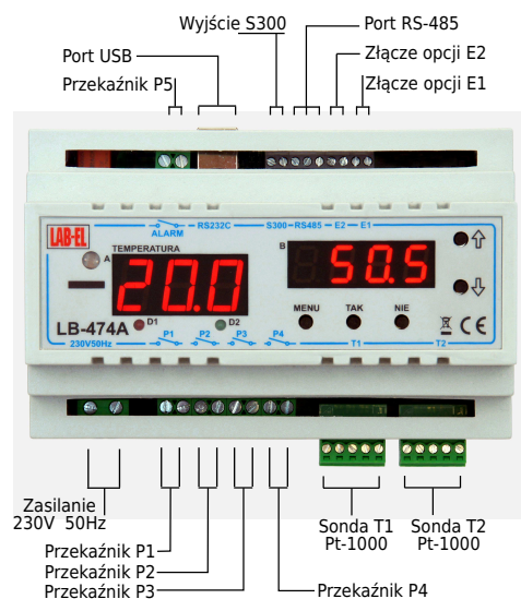
Figure 1: LB-474A3 – punkty wejść i wyjść
