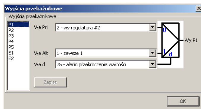
Figure 14: Konfiguracja wyjścia binarnego w programie ws474.exe
