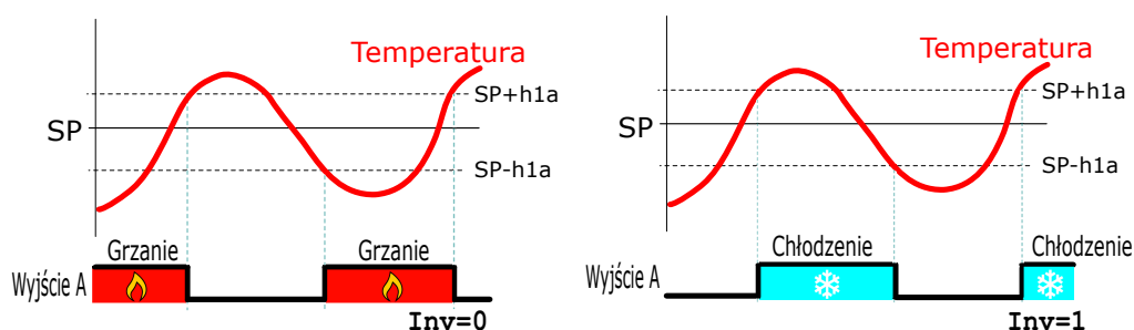
Figure 9: Regulacja progowa, opcja 0 – praca z jednym urządzeniem wykonawczym: po lewej praca z grzałką ( Inv =0), po prawej praca z agregatem chłodniczym ( Inv =1).
