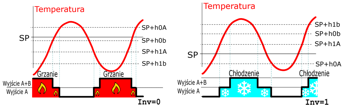
Figure 10: Regulacja progowa, opcja 1 – praca z jednym urządzeniem wykonawczym umożliwiającym stopniowanie mocy. Po lewej sterowanie grzałką ( Inv = 0) ; po prawej sterowanie agregatem chłodniczym ( Inv = 1).
