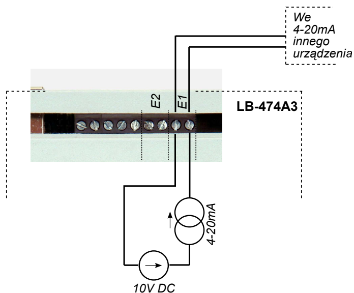
Figure 17: Wyjście 4-20 mA z LB-474A3 dołączone do wejścia odbiornika.
