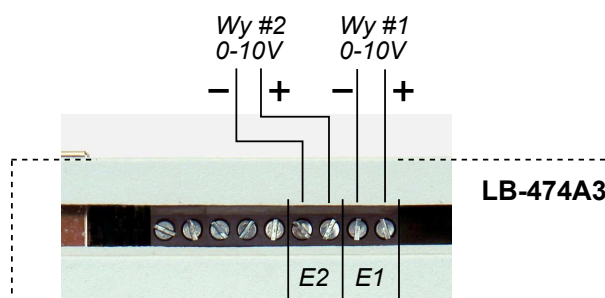
Figure 16: Polaryzacja sygnałów wyjść analogowych 0-10 V
