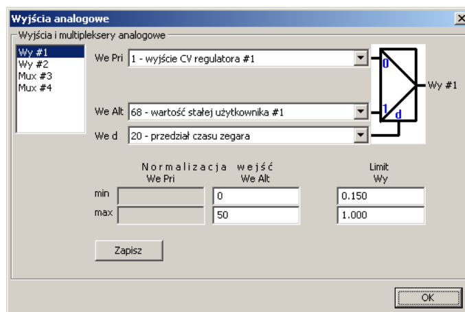
Figure 15: Konfiguracja wyjścia analogowego #1 w programie ws474.exe
