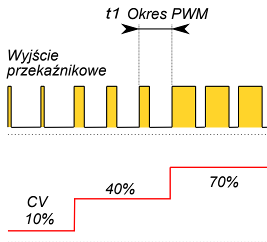
Figure 13: Wyjście algorytmu PID – PWM na przełączniku
