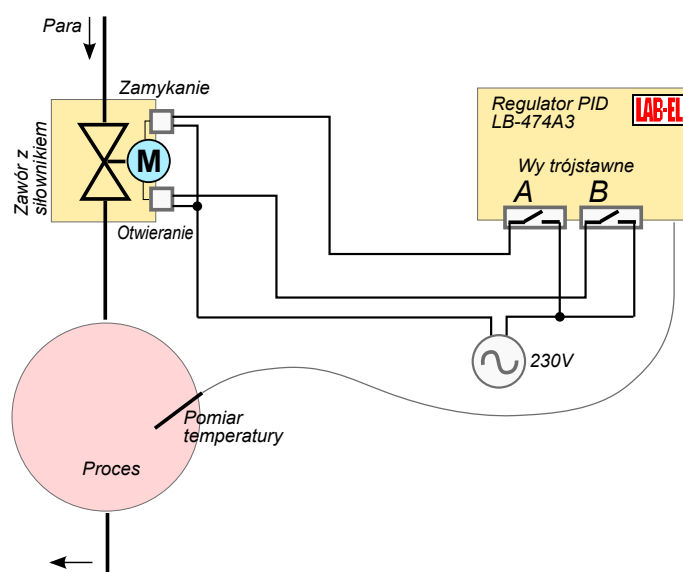
Figure 12: Realizacja PID z wyjściem trójstawnym – regulacja temperatury w obiekcie ogrzewanym parą
