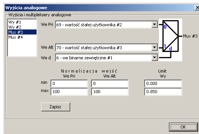
Figure 19: Konfiguracja multiplexera #3 w programie ws474.exe
