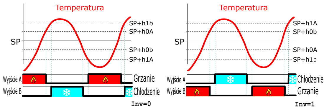
Figure 11: Regulacja progowa, opcja 2 – praca z dwoma urządzeniami wykonawczymi.
