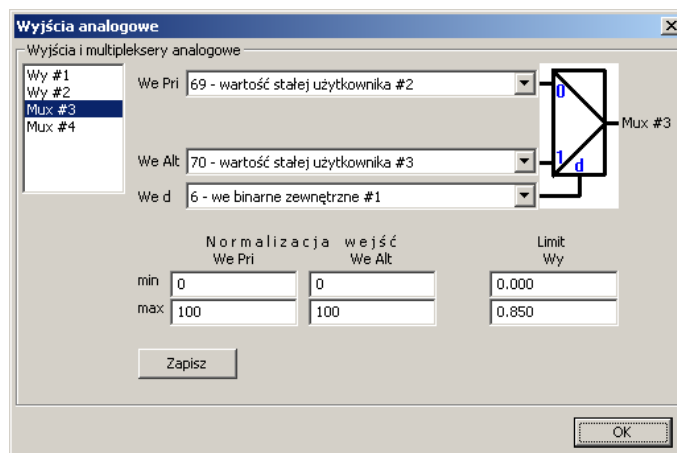
Rysunek 20: Konfiguracja multipleksera #3 w programie ws474.exe
