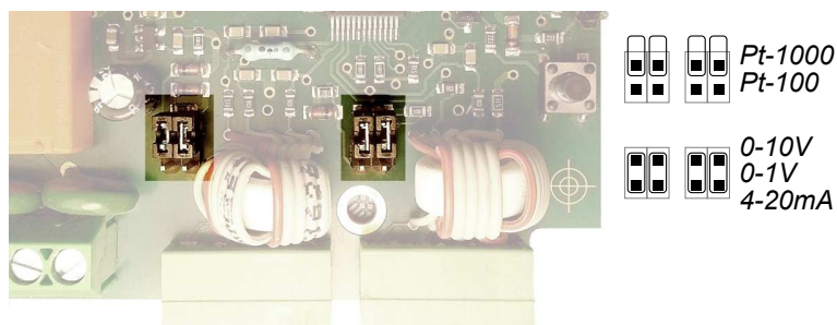
Rysunek 6: Zwory do ustawiania rodzaju wejść – dostępne po otwarciu urządzenia
