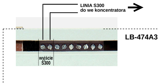
Rysunek 23: Wyjście cyfrowej pętli prądowej S300
