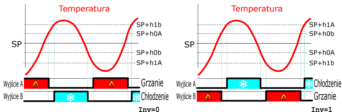
Rysunek 12: Regulacja progowa, opcja 2 – praca z dwoma urządzeniami wykonawczymi.
