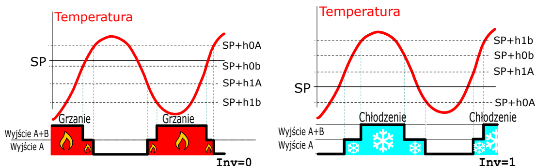
Rysunek 11: Regulacja progowa, opcja 1 – praca z jednym urządzeniem wykonawczym umożliwiającym stopniowanie mocy. Po lewej sterowanie grzałką ( Inv=0 ) ; po prawej sterowanie agregatem chłodniczym ( Inv=1 ).
