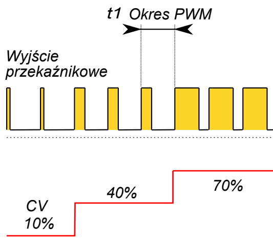
Rysunek 14: Wyjście algorytmu PID – PWM na przełączniku
