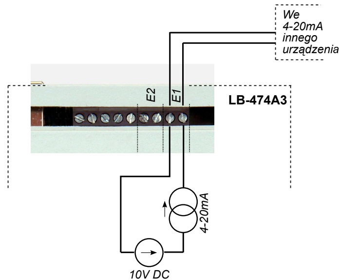
Rysunek 18: Wyjście 4-20 mA z LB-474A3 dołączone do wejścia odbiornika.
