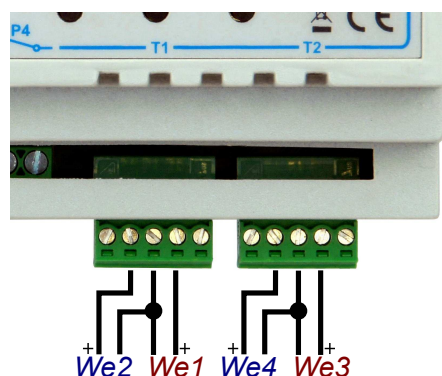
Rysunek 7: Numeracja wejść w konfiguracji napięciowej
