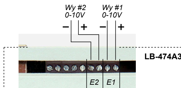
Rysunek 17: Polaryzacja sygnałów wyjść analogowych 0-10 V
