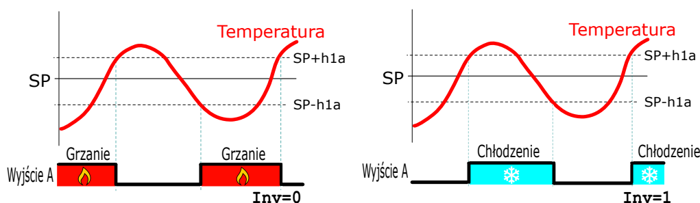
Rysunek 10: Regulacja progowa, opcja 0 – praca z jednym urządzeniem wykonawczym: po lewej praca z grzałką ( Inv = 0), po prawej praca z agregatem chłodniczym ( Inv = 1).
