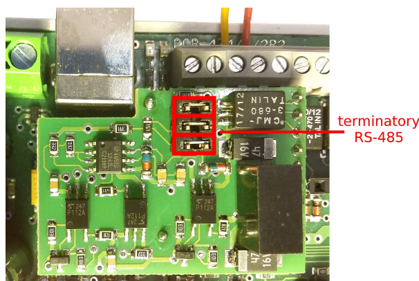
Rysunek 22: Jumpery (zworki) terminatorów opcjonalnego portu RS-485
