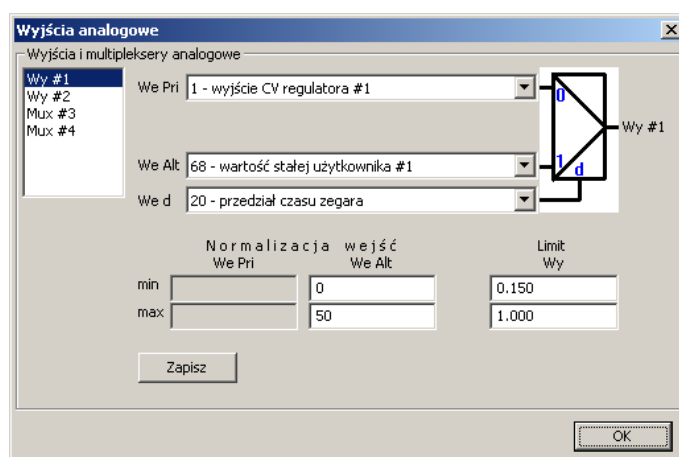
Rysunek 16: Konfiguracja wyjścia analogowego #1 w programie ws474.exe
