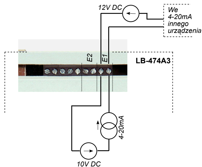
Rysunek 19: Wyjście 4-20 mA z LB-474A3 z dodatkowym źródłem zasilania pętli (12 V DC), dołączone do wejścia odbiornika.
