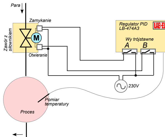
Rysunek 13: Realizacja PID z wyjściem trójstawnym – regulacja temperatury w obiekcie ogrzewanym parą
