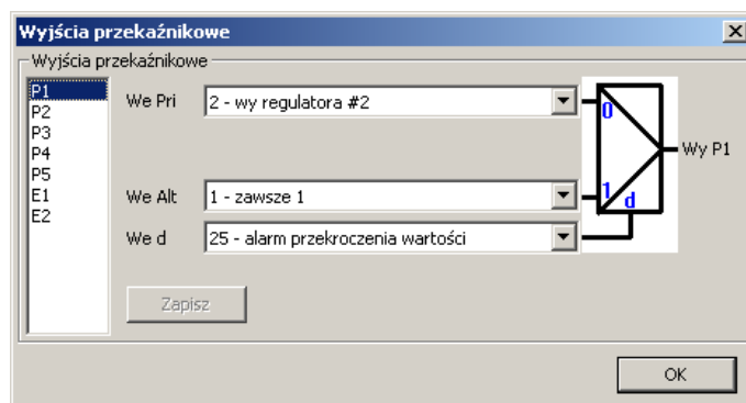
Rysunek 15: Konfiguracja wyjścia binarnego w programie ws474.exe
