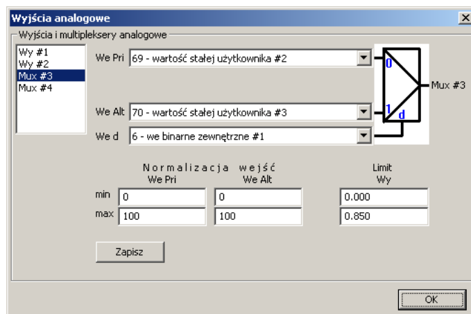
Rysunek 20: Konfiguracja multipleksera #3 w programie ws474.exe
