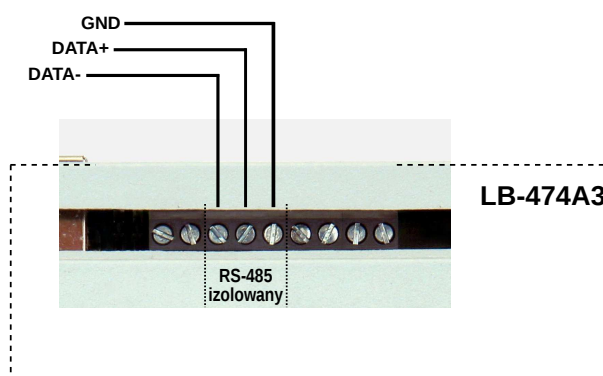
Rysunek 21: Wyjście opcjonalnego interfejsu RS-485
