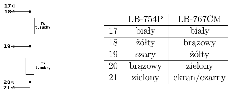
Rysunek 2: Sposób przyłączenia sond Pt-1000 oraz opis kolorów przewodów dla psychrometrów LB-754P i LB767CM.
