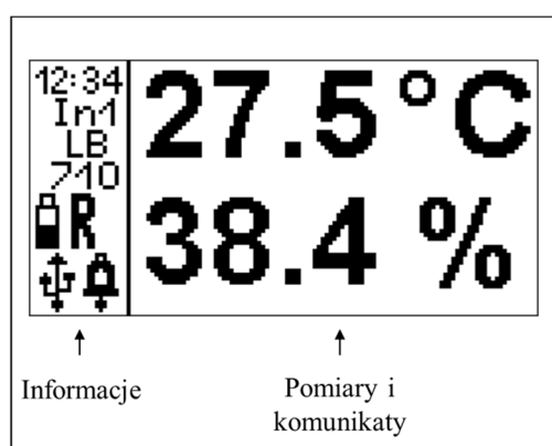
Rys. 2 Wyświetlacz LB-757
